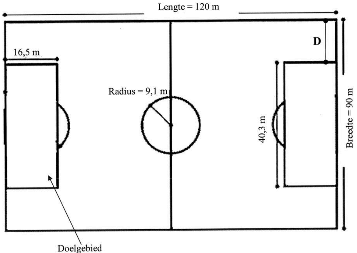
DIAGRAM 1: SOKKERVELD MET WERKLIKE AFMETINGS
