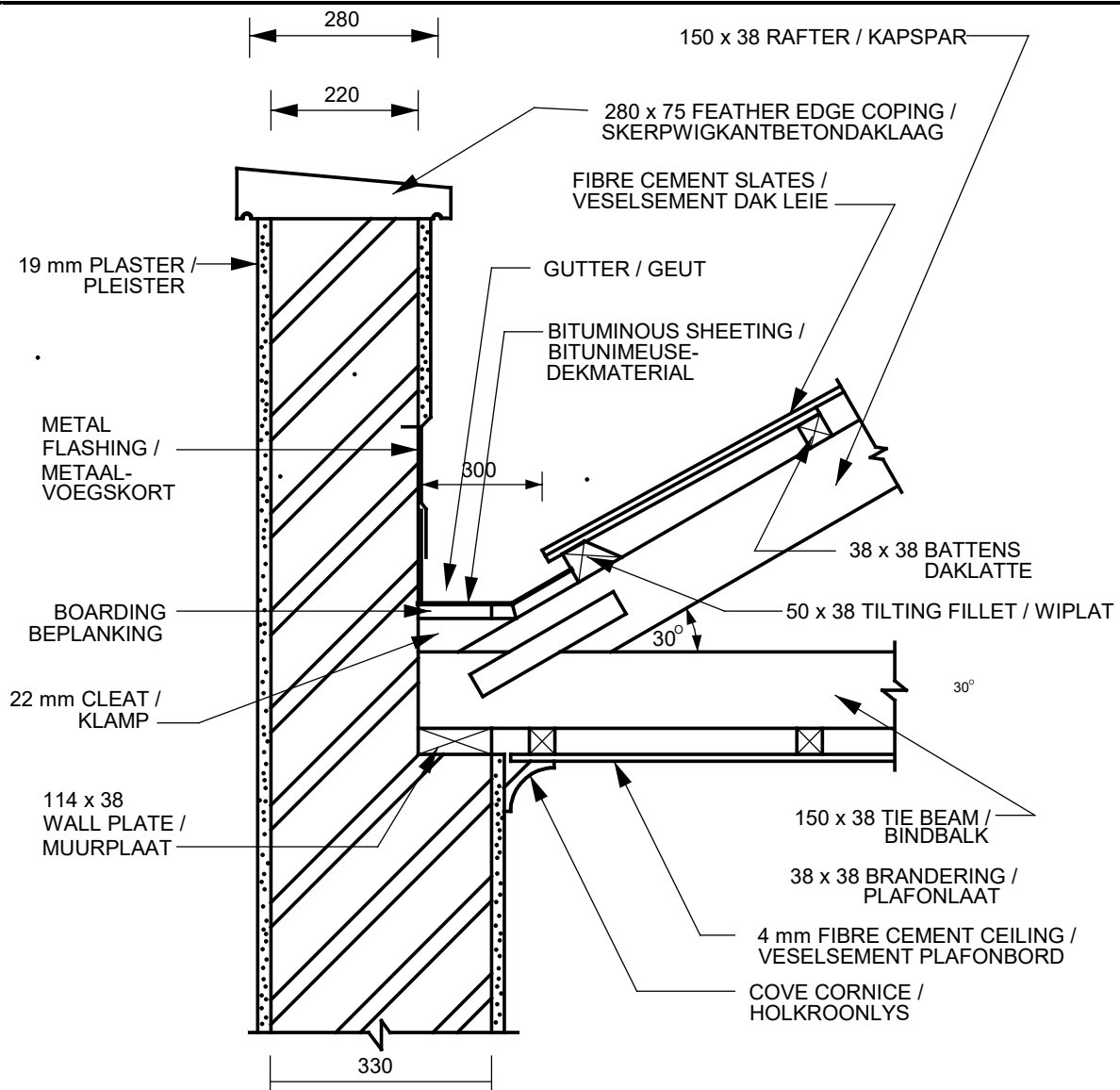
VERTIKALE DEURSNEE DEUR 'N BORSWERINGGEUT SKAAL 1 : 10
