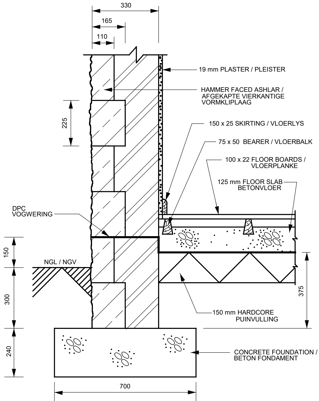
VERTIKALE DEURSNEE DEUR KLIPMUUR SKAAL 1 : 10
