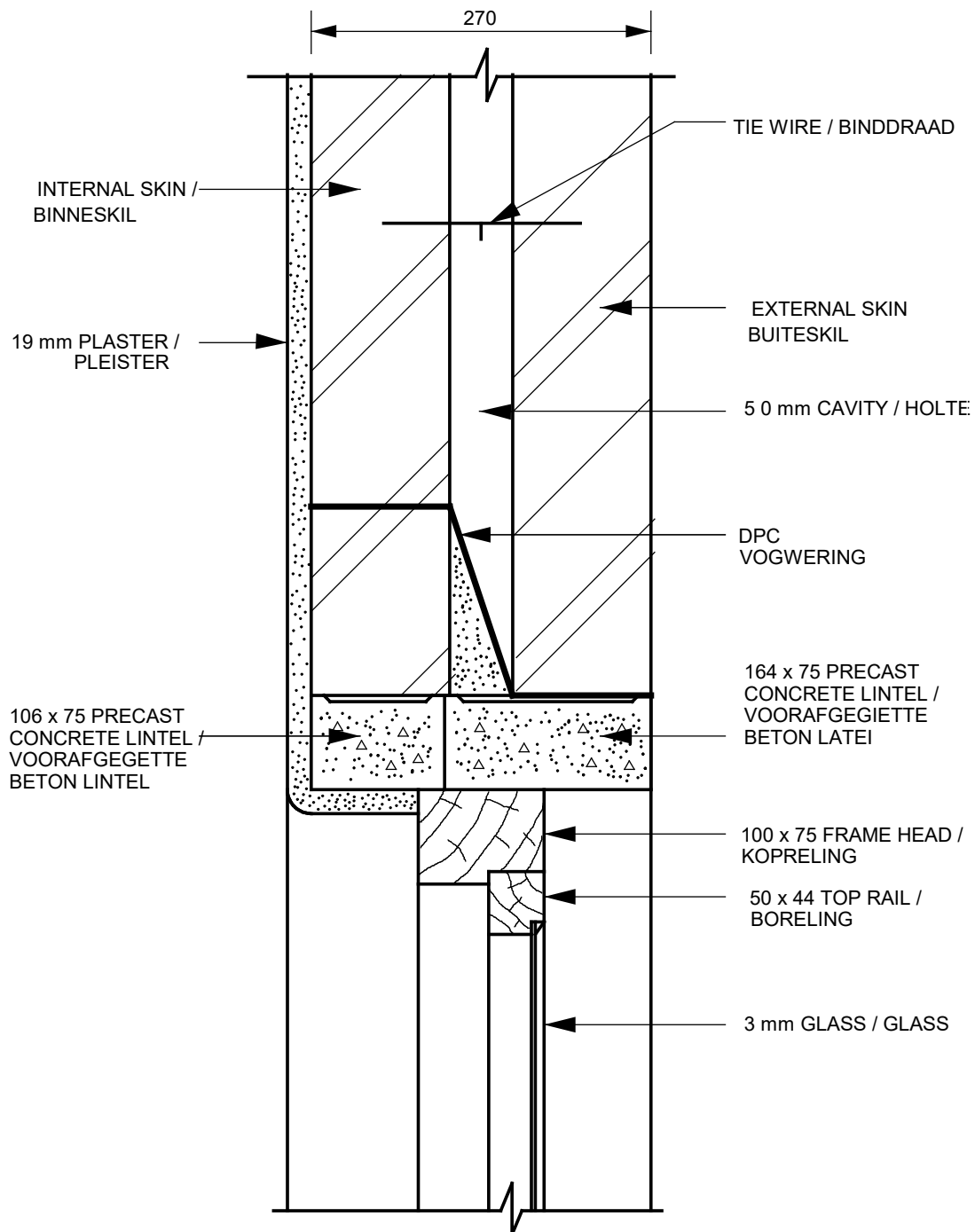
VERTIKALE DEURSNEE DEUR DIE BOKANT VAN RAAM EN VOORAF GEGOTE BETONLATEI SKAAL 1 : 5
